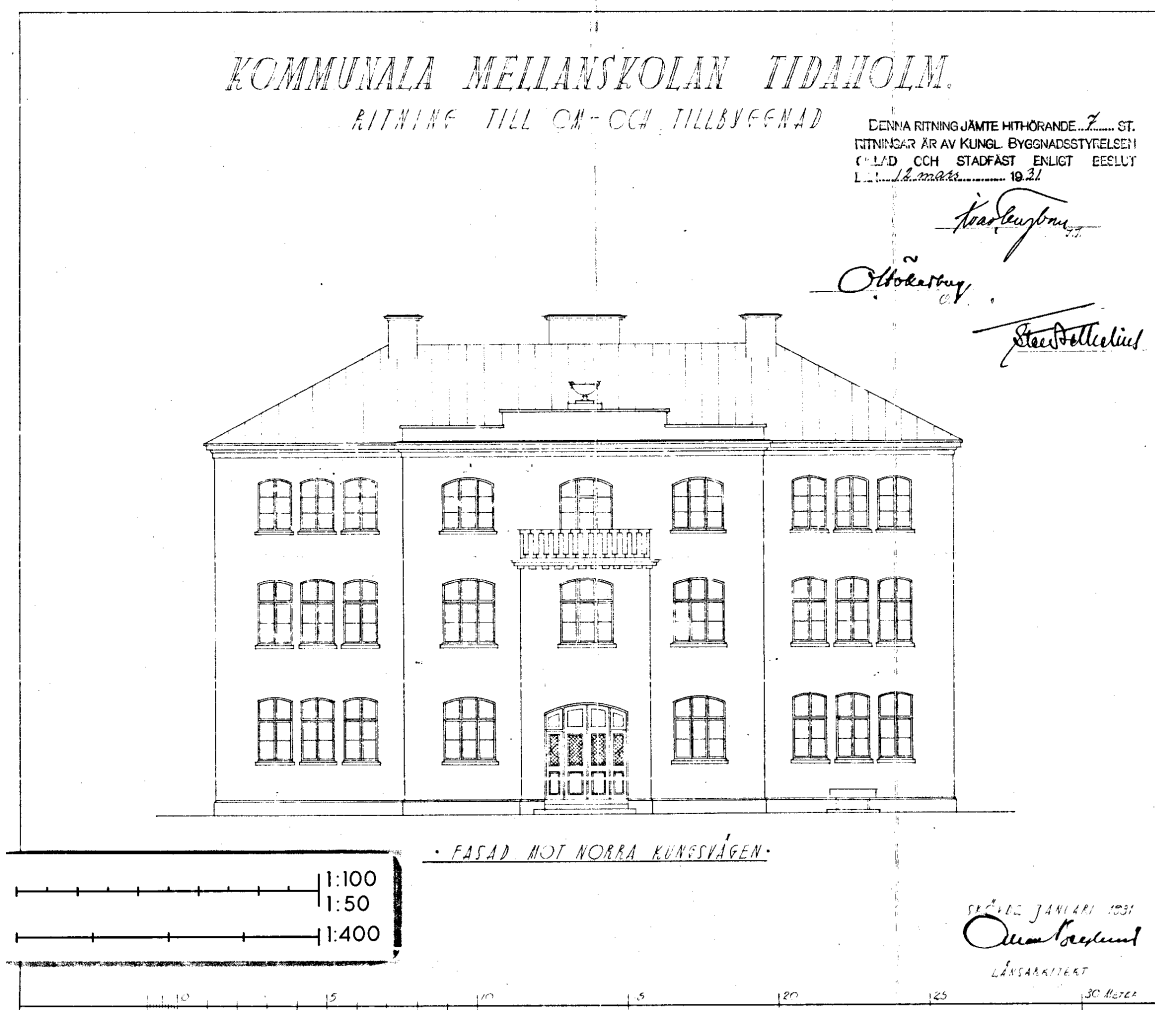
Länssarkitekt Allan Berglunds ritning till om- och tillbyggnad, 1931. Fasad mot Norra Kungsvägen. Byggnadsnämndens arkiv, Tidaholms kommun.
